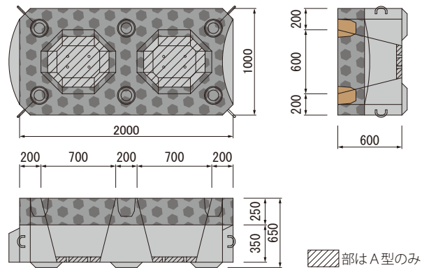
製品図
