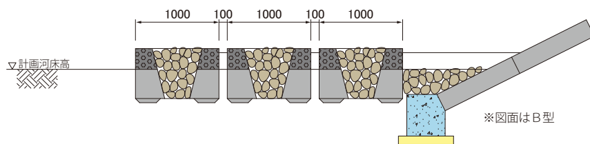
標準断面図
